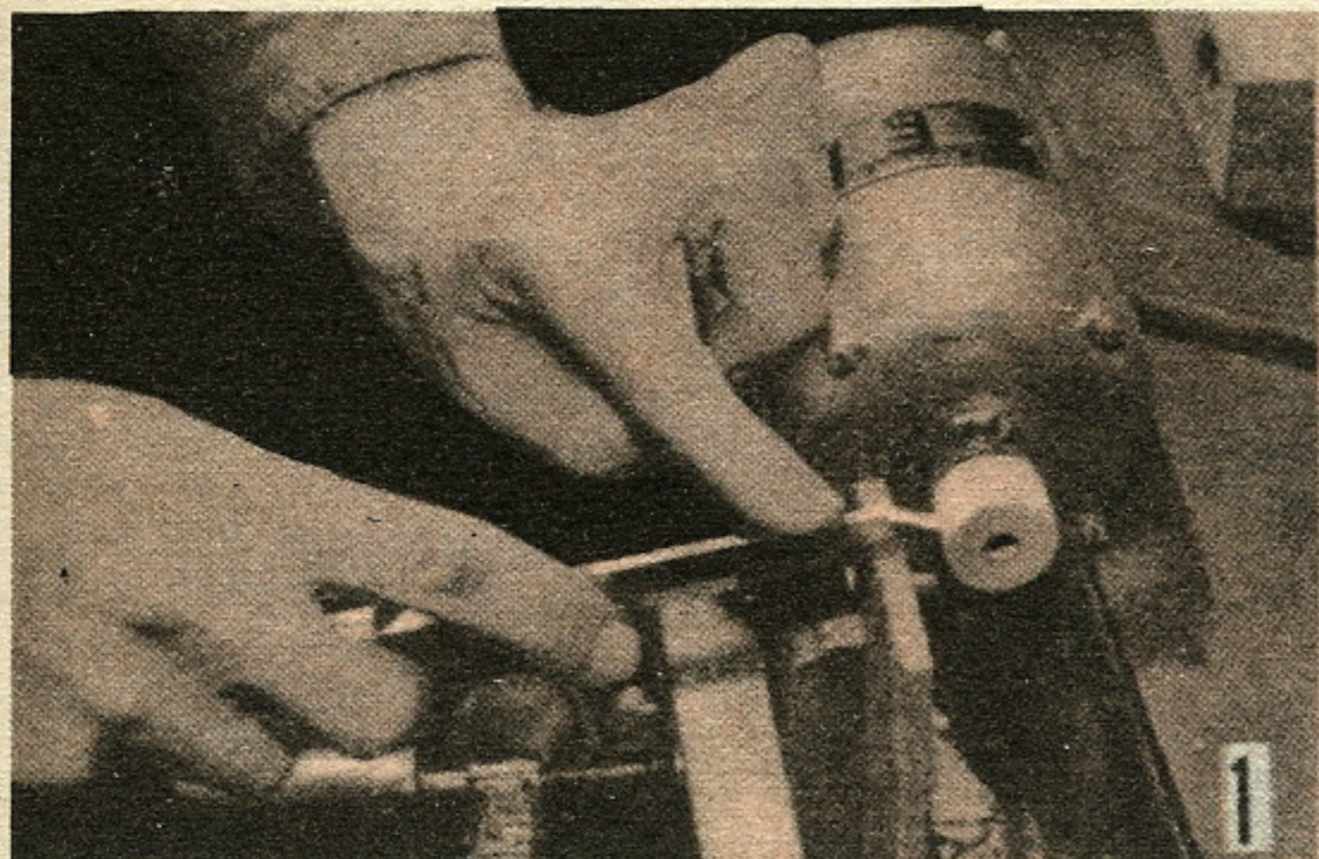
(Foto a sinistra): Tornitura del cilindretto o puleggina ad attrito che si trova sull'asse rotante del motore elettrico; si tratta di fare nel cilindretto, una gola molto larga e poco profonda in modo da aumentare la presa del cilindretto sul volantino della macchina da cucire. — (Foto a destra): Molletta di filo di acciaio, che serve ad allontanare il complesso dalla macchina quando si intende fermare la macchina stessa. Quando il pedale viene premuto, viene vinta la resistenza di questa molla ed il complesso si trova a ridosso del volantino in modo che il cilindretto sull'asse del motore possa trasmettere ad esso il movimento.
