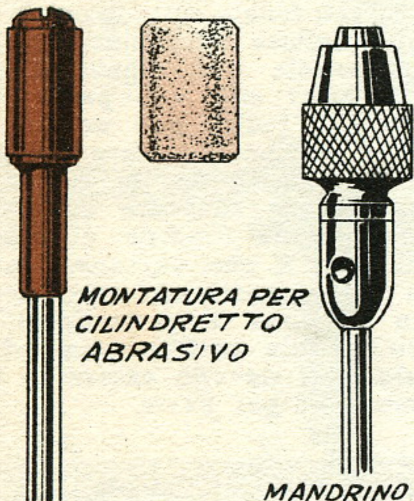
TIPICHE FRESETTE DA INCISORE
